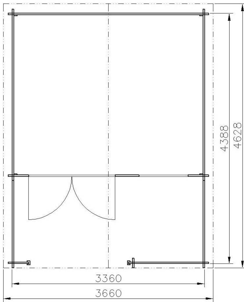
PŮDORYS
