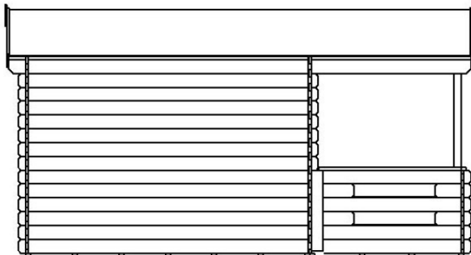
BOČNÍ STĚNA LEVÁ C
