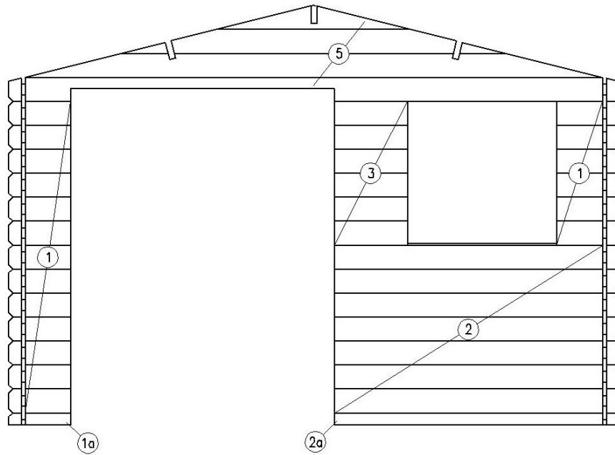
PŘEDNÍ STĚNA A
