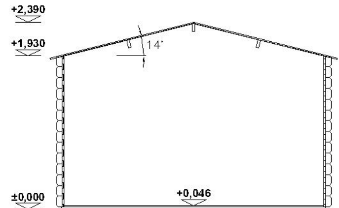
ŘEZ
