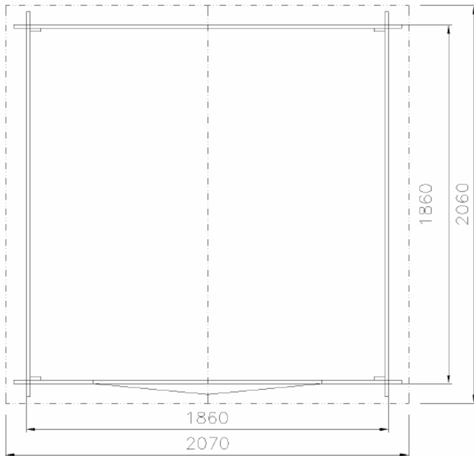
PŮDORYS
