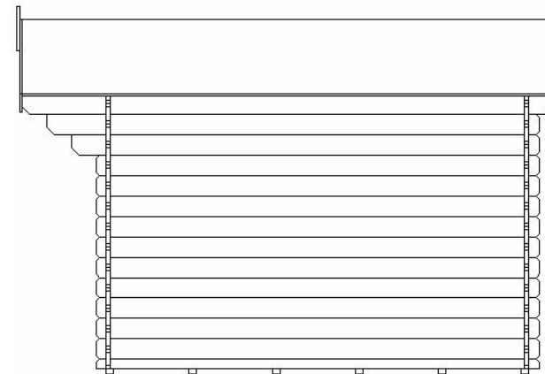
ŘEZ
