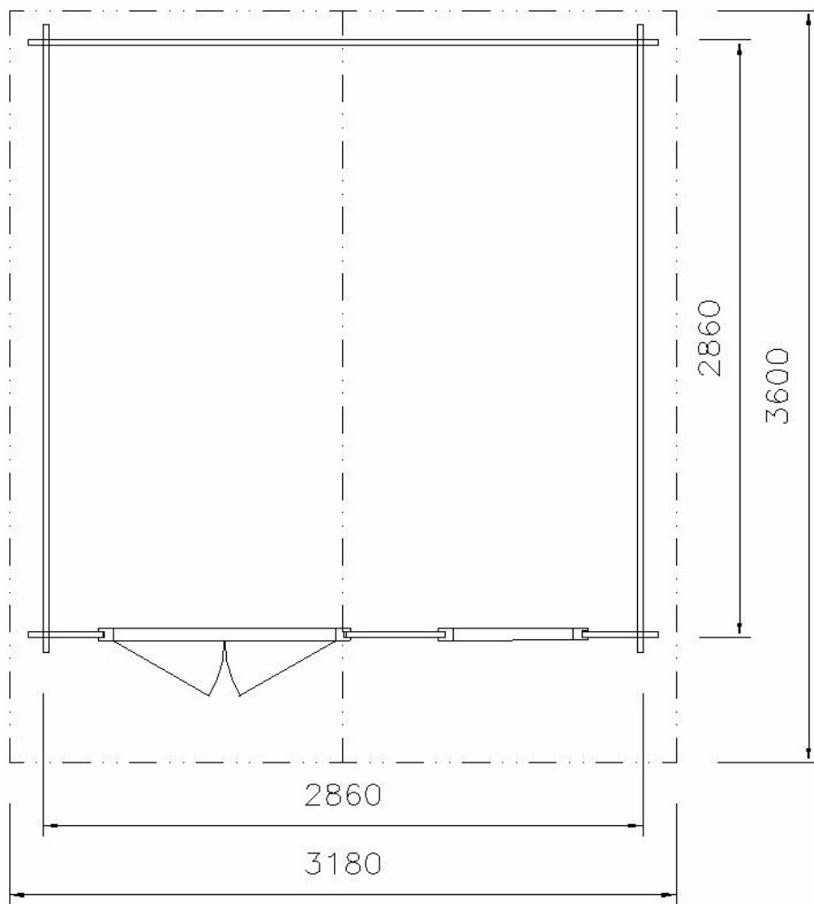
PŮDORYS
