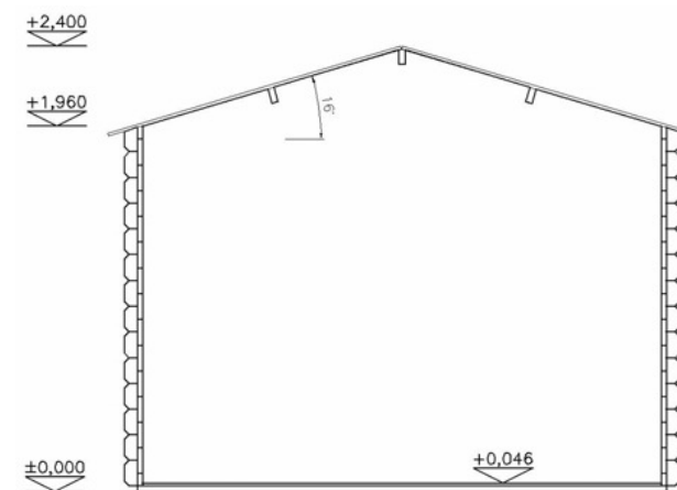
ŘEZ
