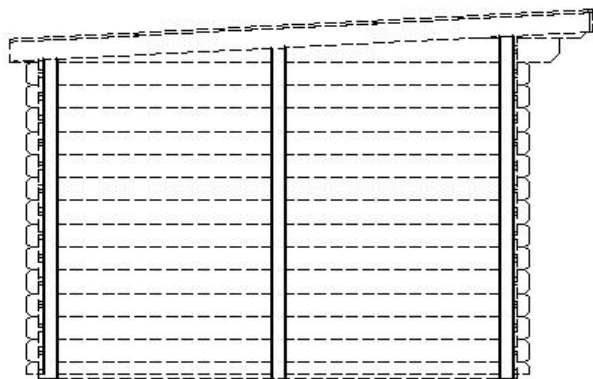
BOČNÍ STĚNA LEVÁ C
