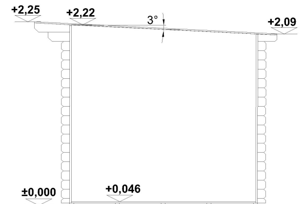
ŘEZ
