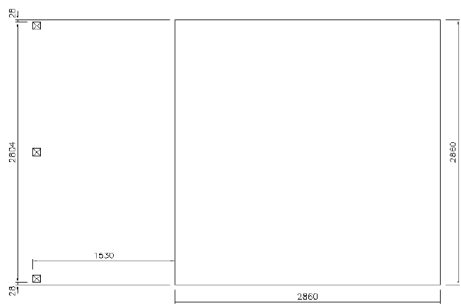
ROZMĚRY ZÁKLADOVÉ DESKY
