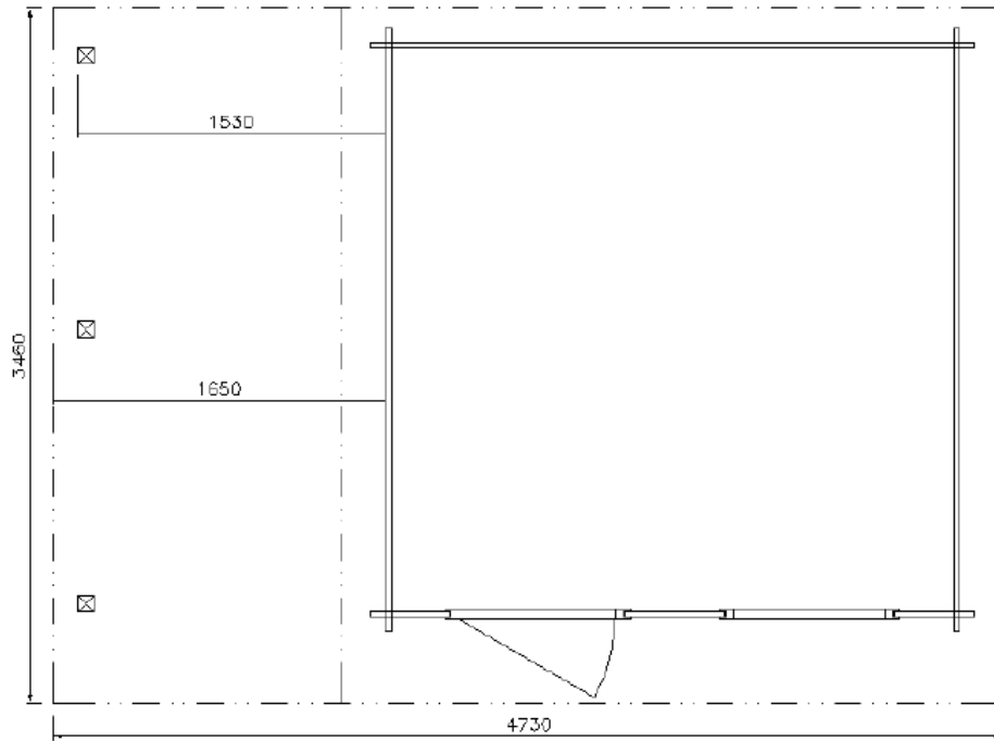
PŮDORYS
