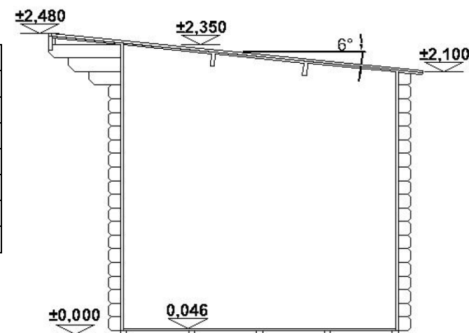
ŘEZ
