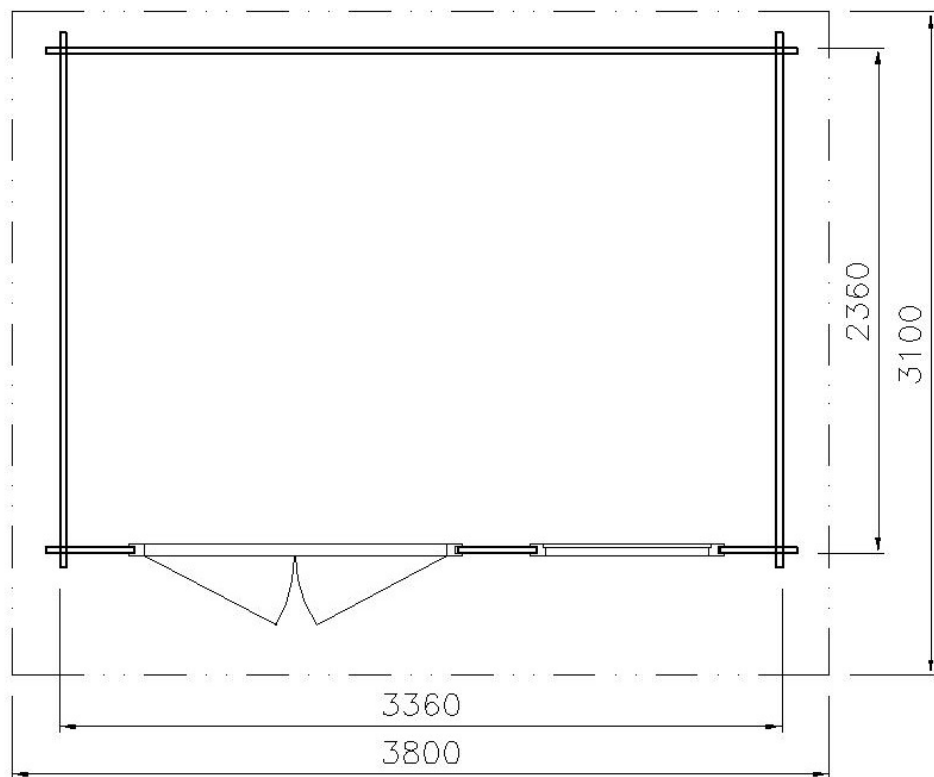
PŮDORYS
