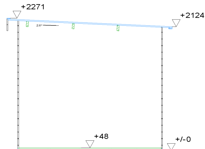
ŘEZ
