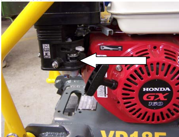
Obr. Otevřený palivový kohout motoru
