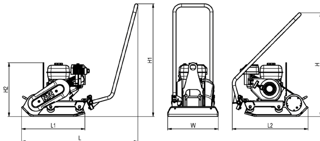
Obr. Základní popis stroje
