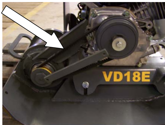
Obr. Kontrola napnutí klínového řemenu
