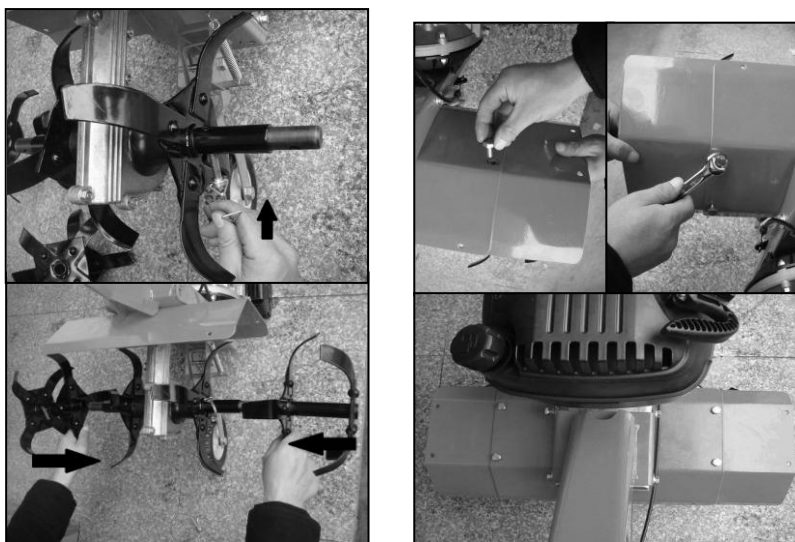
Montáž nožů a krytu kultivátoru
