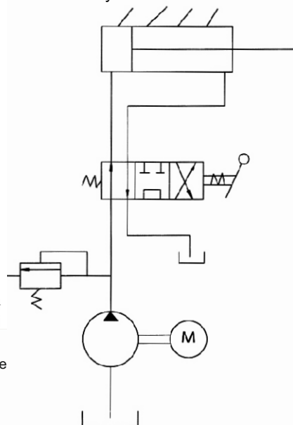
hydraulické schéma
