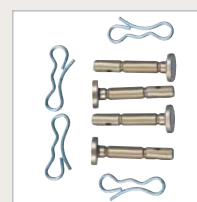
SADA 4 STŘIŽNÝCH ŠROUBŮ A ZÁVLAČEK PRO DVOUSTUPŇOVÉ SNĚHOVÉ FRÉZY MTD OBJEDNACÍ ČÍSLO: 7011-M6-0010
